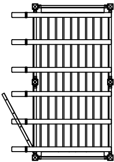
DTP-5 TOP VIEW N.T.S.
