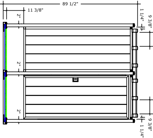
DTP-5 ELEVATION N.T.S.
